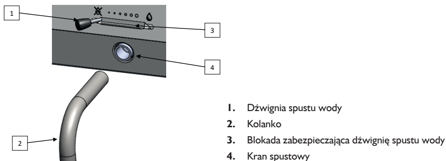
Rys. 9. Elementy mechanizmu spustowego wody
