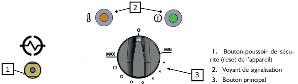
Fig. 8. Eléments du panneau de commande
