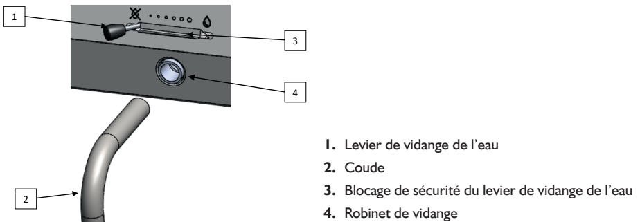
Fig. 9. Eléments du mécanisme de vidange de l'eau
