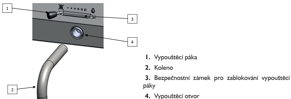
Obrázek č. 9. Prvky mechanismu pro vypouštění vody
