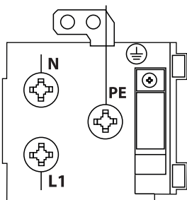
Figure 7. Branchement de l'appareil au réseau électrique
