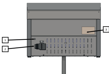
Fig. 5. Raccordement de l'appareil à une installation équipotentielle.
