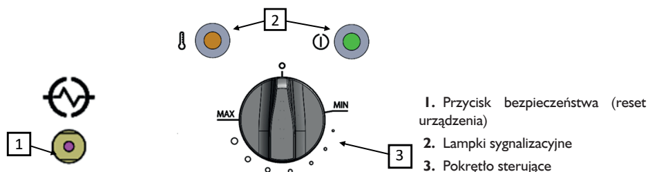
Rys. 8. Elementy sterujące urządzenia
