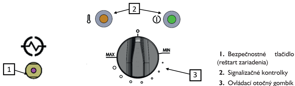
Obrázok 8. Ovládacie prvky zariadenia
