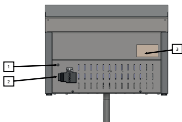
Figura 5. Conexión del equipo a una instalación equipotencial.
