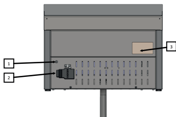
Obrázek č. 5. Připojení přístroje k zařízení pro vyrovnávání potenciálu.
