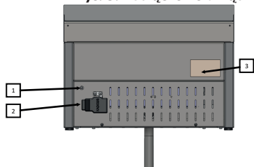
Rys. 5. Podłączenie urządzenia do instalacji wyrównującej potencjały elektryczne.
