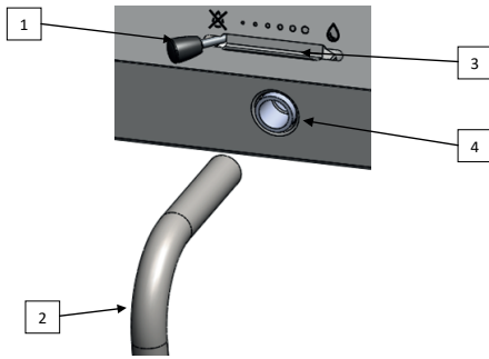
Bild 9. Elemente des Mechanismus des Wasserablassens
