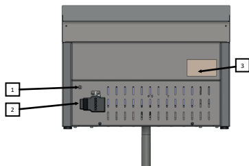
Obrázok 6. Pohľad na zariadenie zo zadnej strany.
