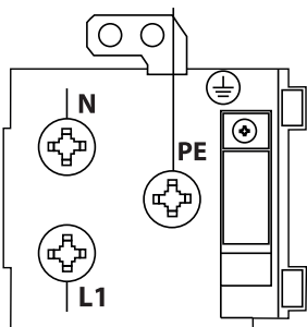
Figura 7. Conexión del equipo a la instalación eléctrica.
